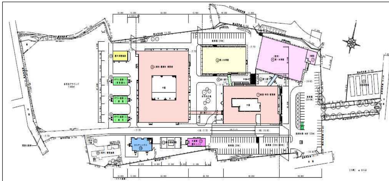
統合校配置計画図
